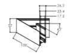
MG-321-20B-M45 Size: 100*76*62mm Material: Aluminum
