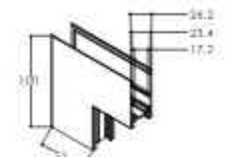
MG-321-20B-MW Size: 100*100*25.8mm Material: Aluminum
