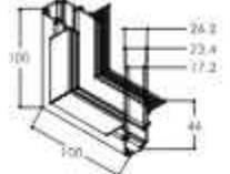
MG-321-20-AL Size: 100*100*46mm Material: Aluminum
